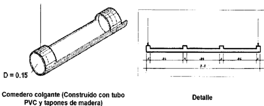
Figura 3. Vista general de un comedero colgante y sus dimensiones
